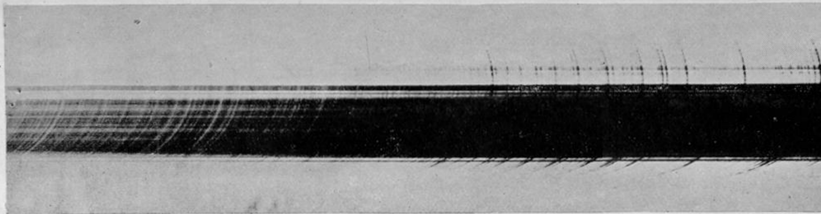
SPECTRUM N° 13. E
