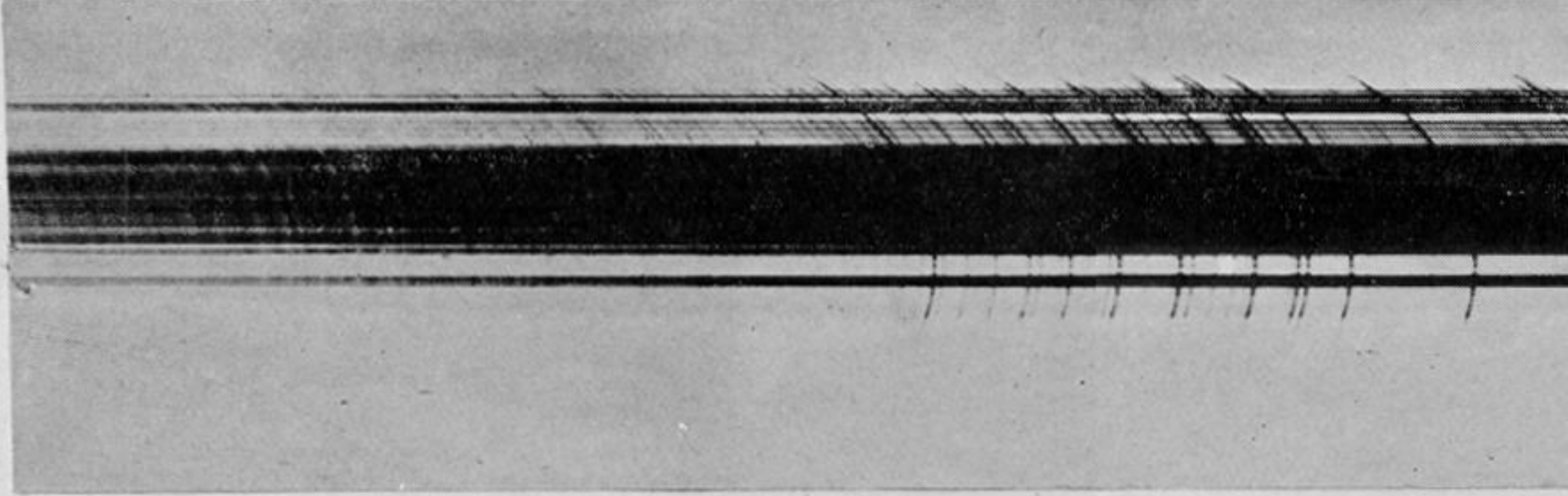
SPECTRUM N° 9. E
